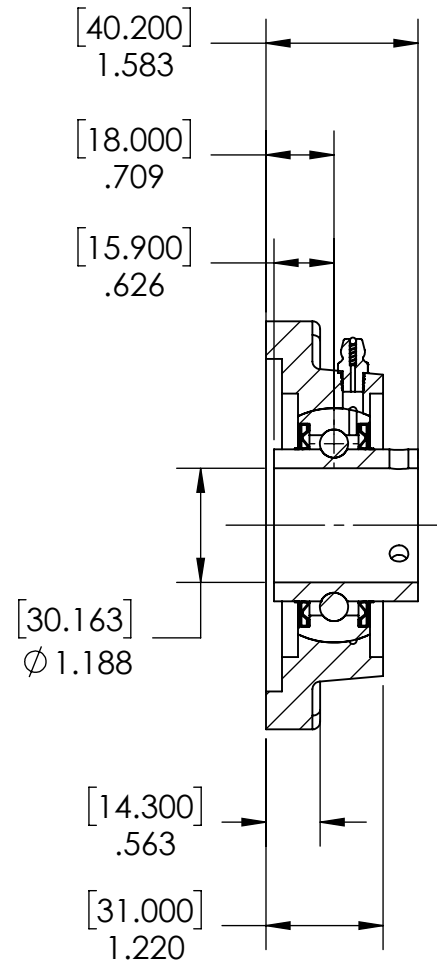
SECTION A-A
